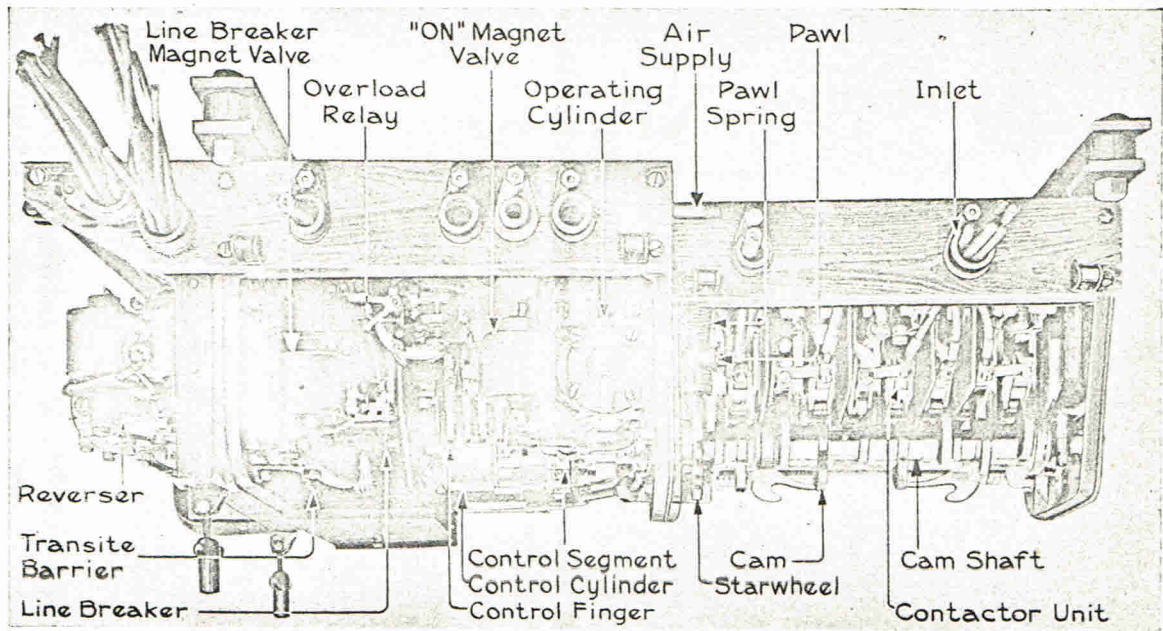
Fig. 30. PC-5 Controller
